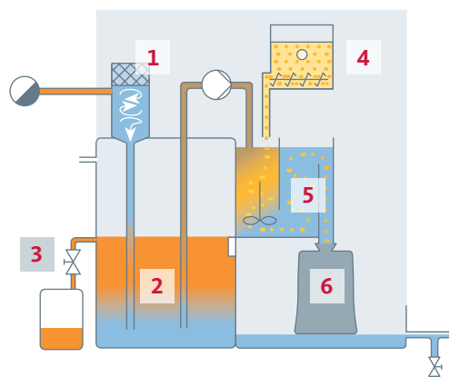
Schema BEKOSPLIT® 11
